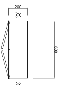
Top elevation
